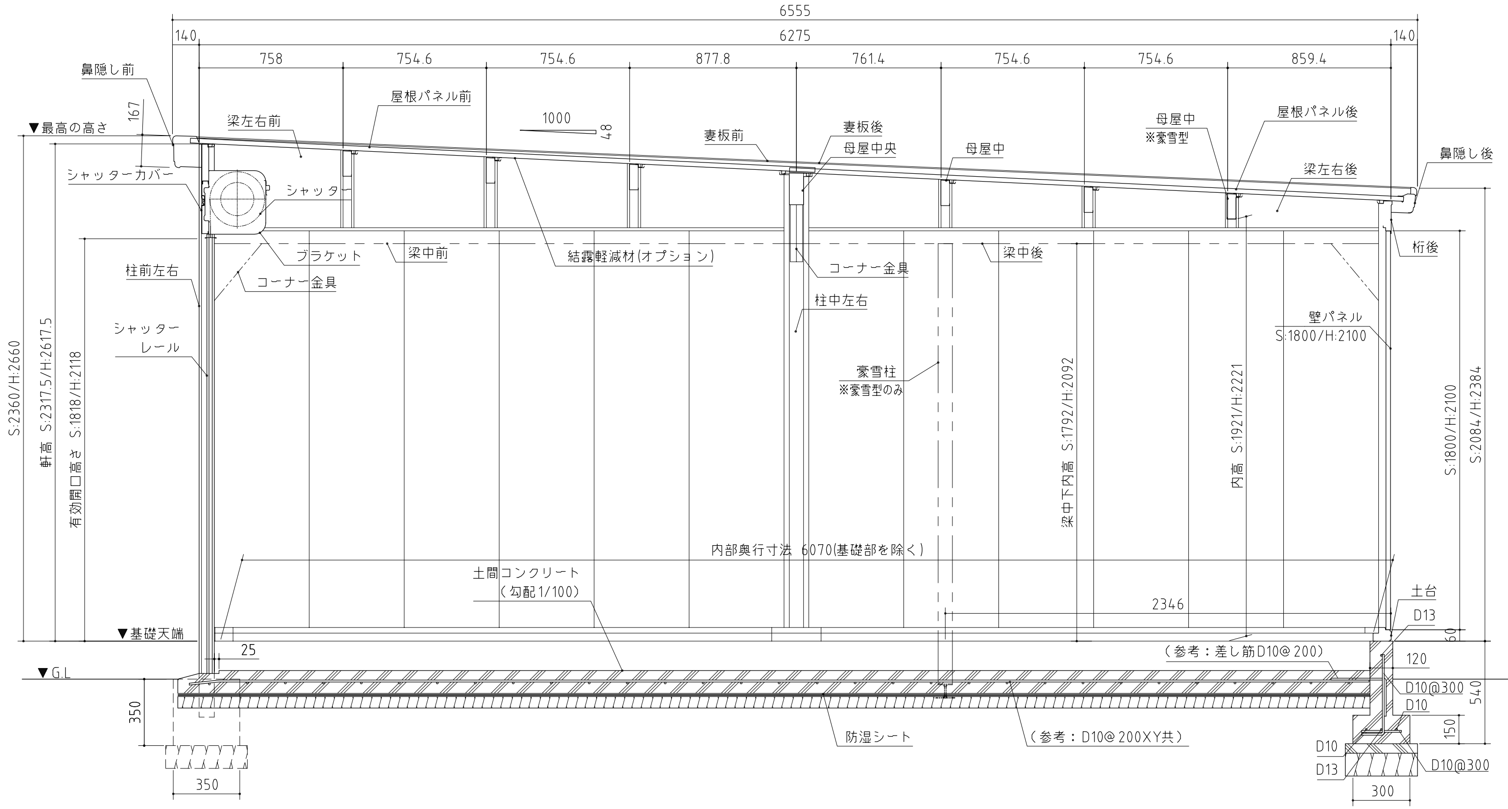
断面図(側面) <縮尺> S=1/20 ~一般型・豪雪型~ 機種名 GRN- 2662S・SL・H・HL、3162S・SL・H・HL 3662S・SL・H・HL
